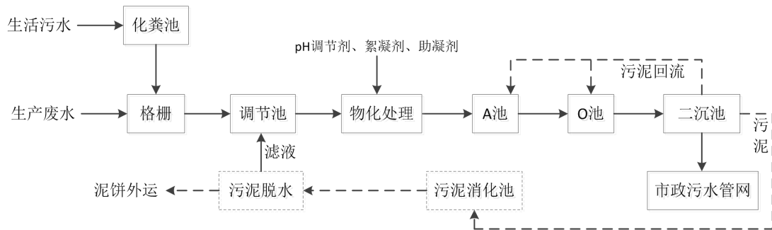
图4-1 厂内污水处理站处理工艺流程图
