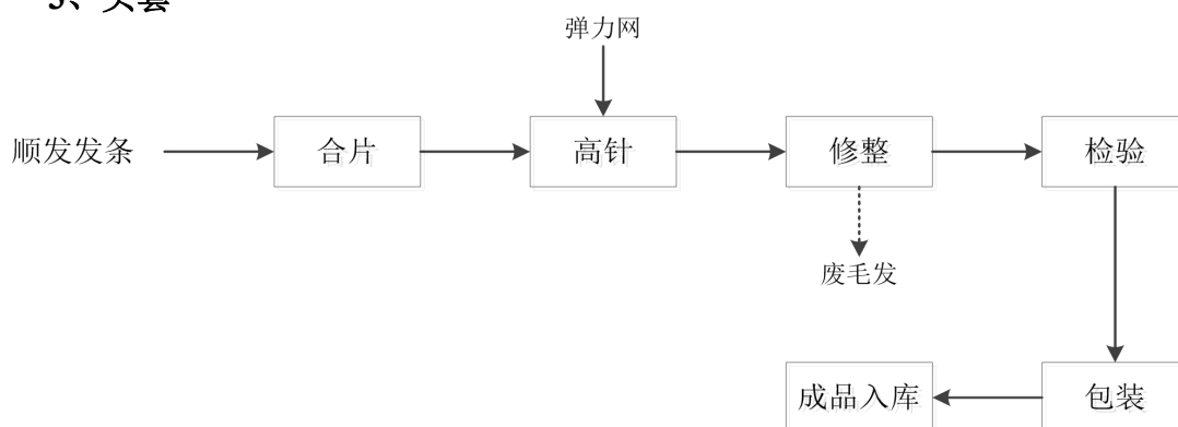
图 2-4 头套生产工艺流程及产污节点图
