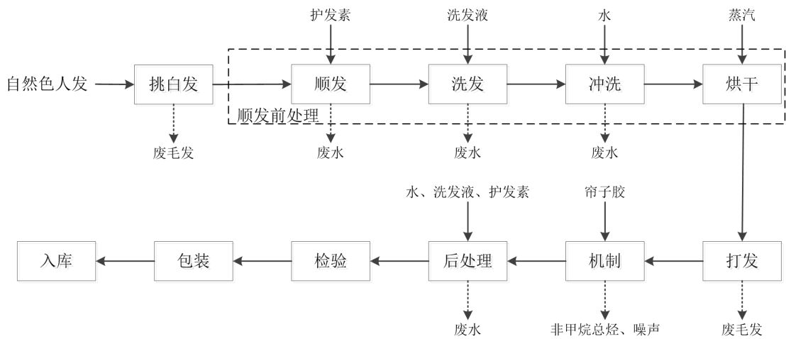
图2-2 顺发发条生产工艺流程及产污节点图
