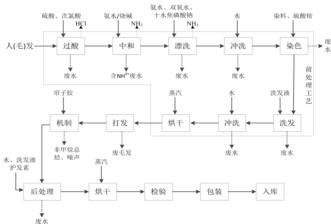
图2-3 泡发发条生产工艺流程及产污节点图
