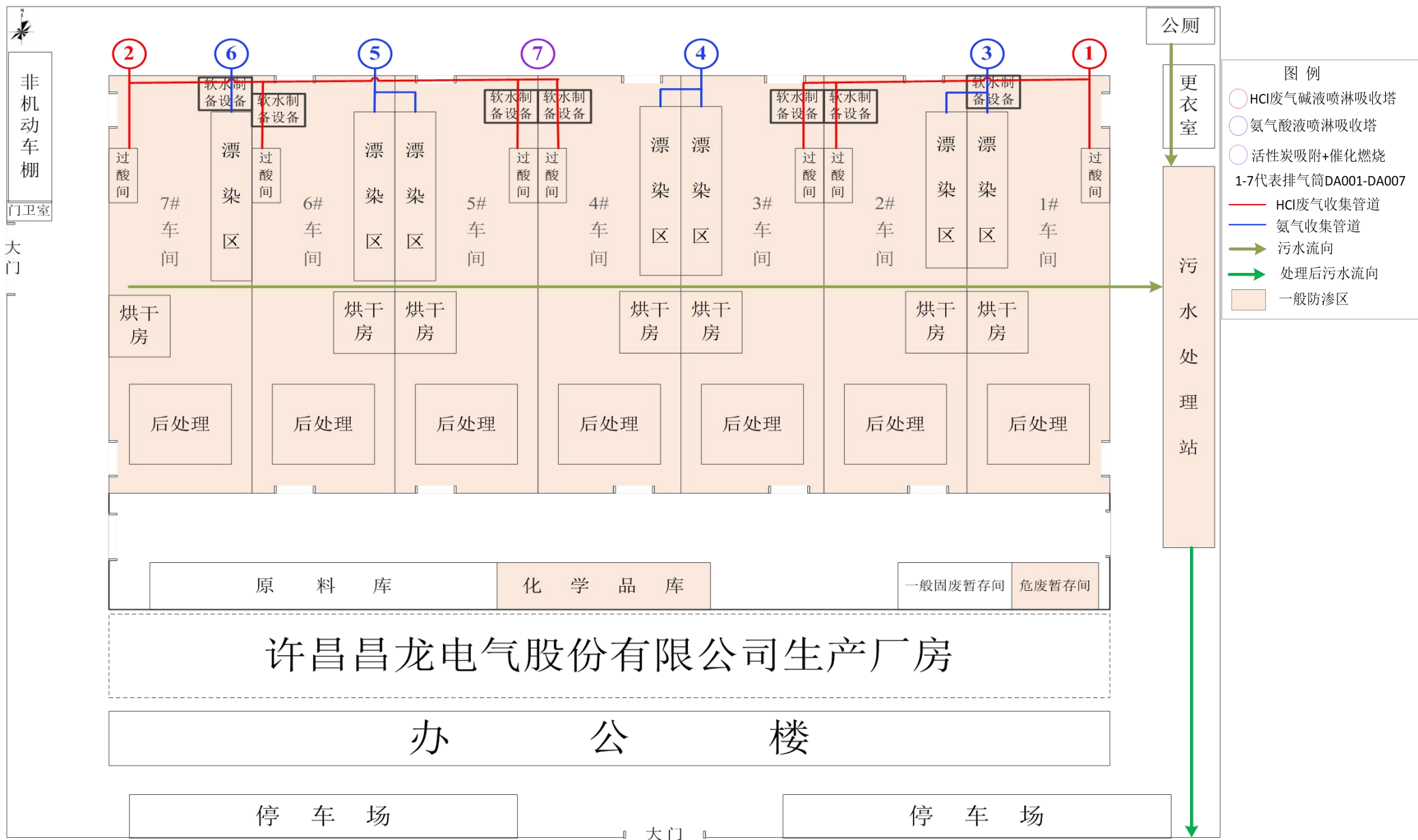
附图三 项目平面布置图（一层）
