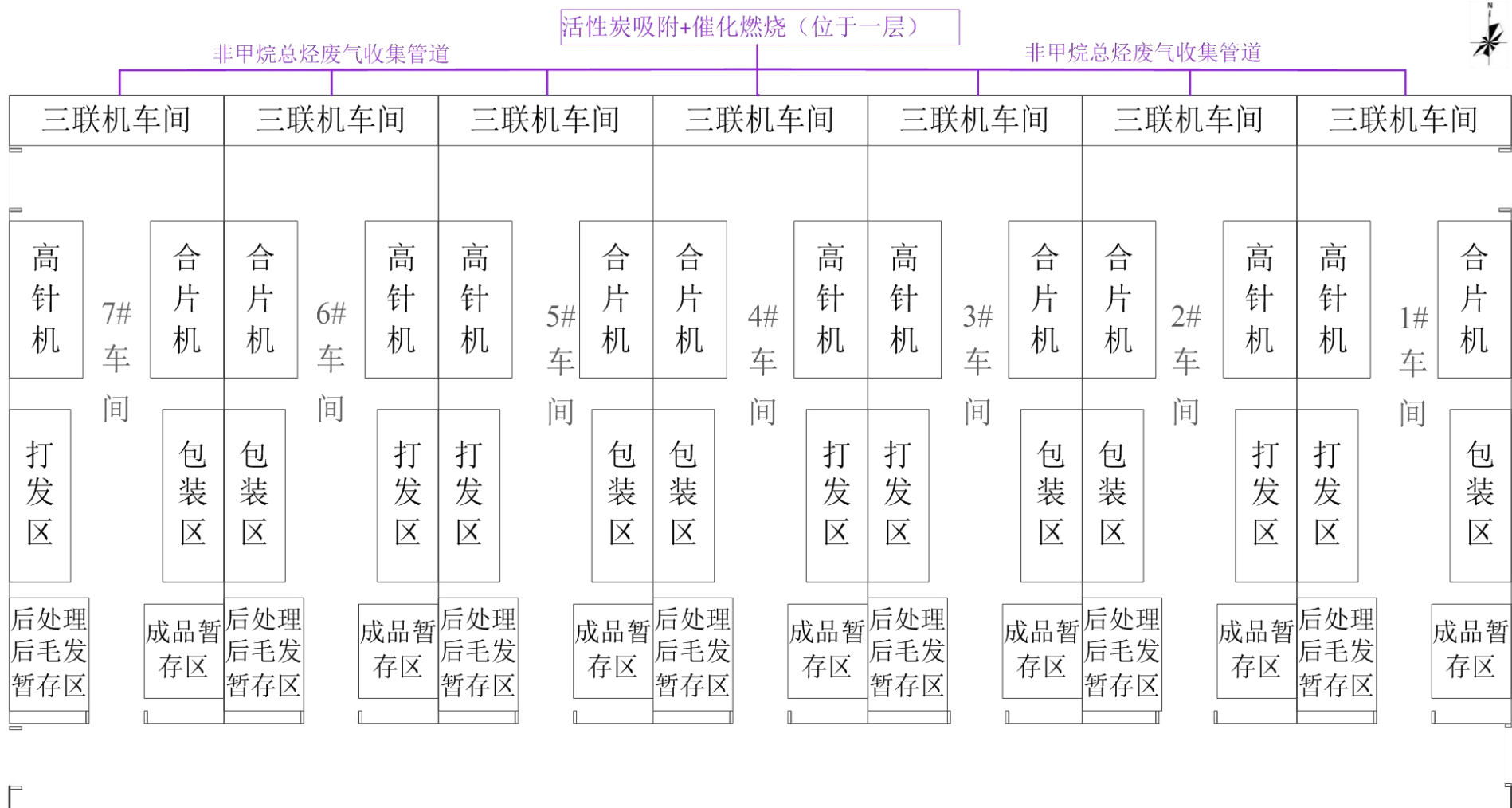
附图四 车间二层平面布置图
