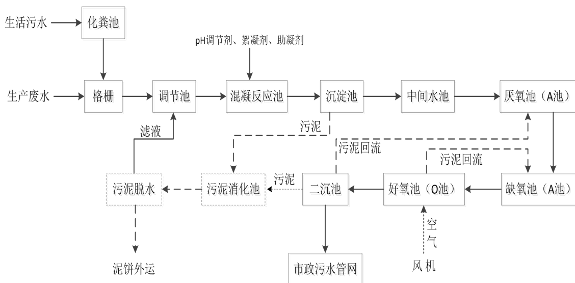
图4-1 厂区污水处理站处理工艺流程图
