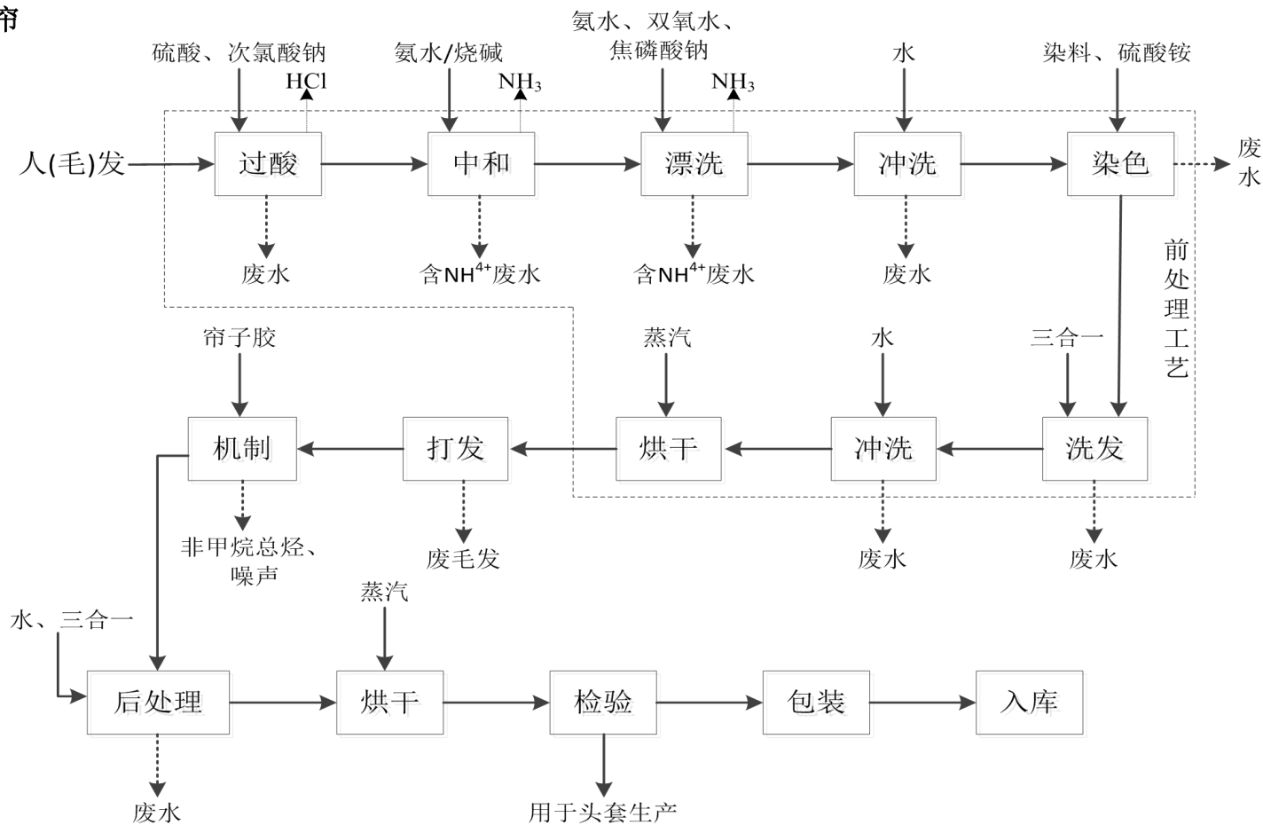
图2-2 发帘生产工艺流程及产污节点图
