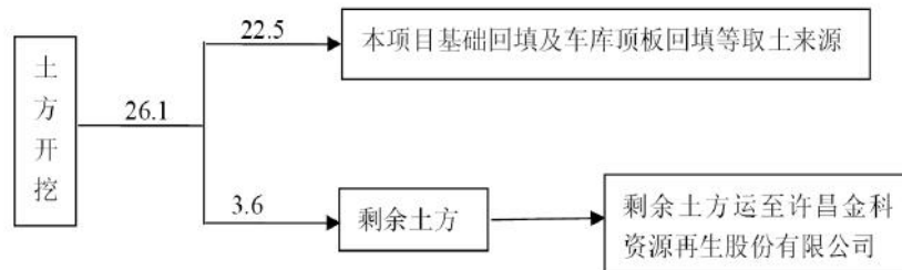
图2 项目土石方平衡 单位：万 m 3
