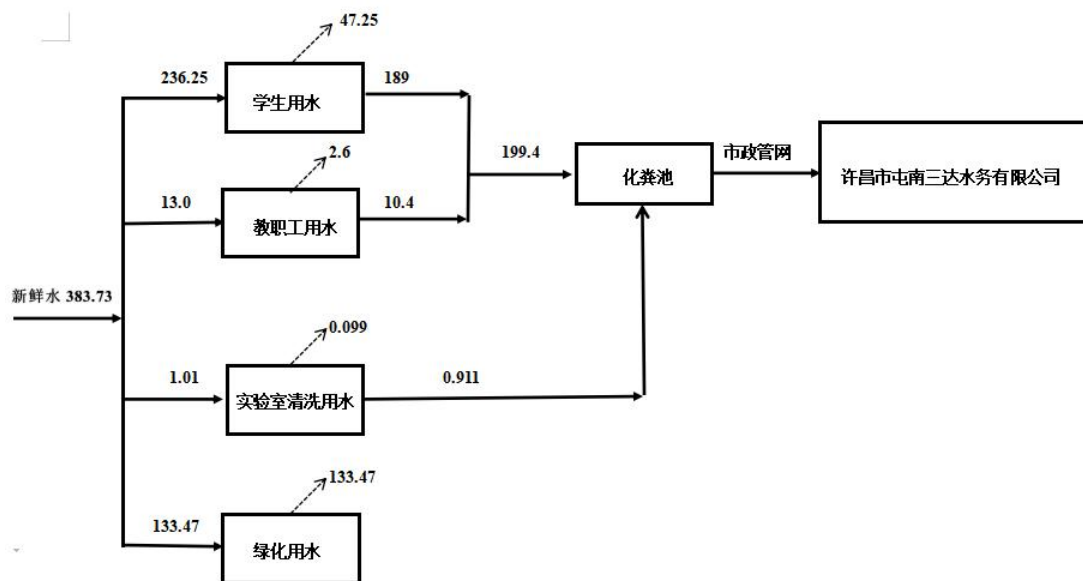
图 3 本项目水平衡图 (m 3 /d)
