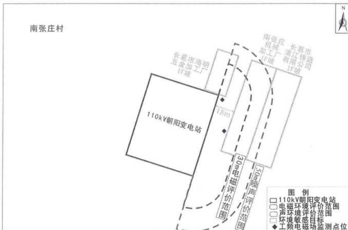
图 2 本项目朝阳变电站周边情况及监测点位示意图
