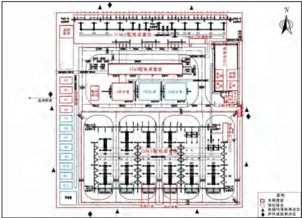
图 3-1 220kV 渔唱变电站监测点位示意图
