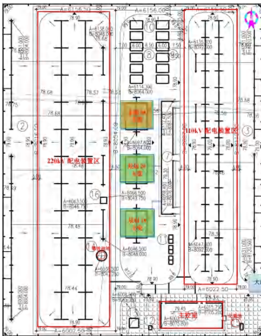
图2-5 220kV 灌台变电站平面布置示意图
