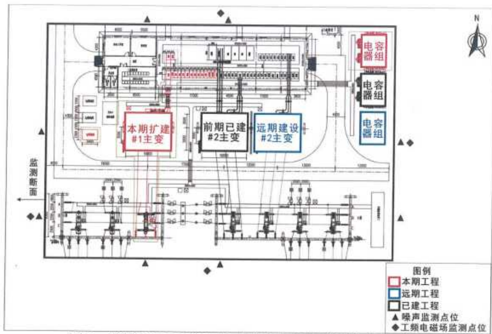
图 1 滨湖 110kV 变电站电磁和声环境监测点位示意图
