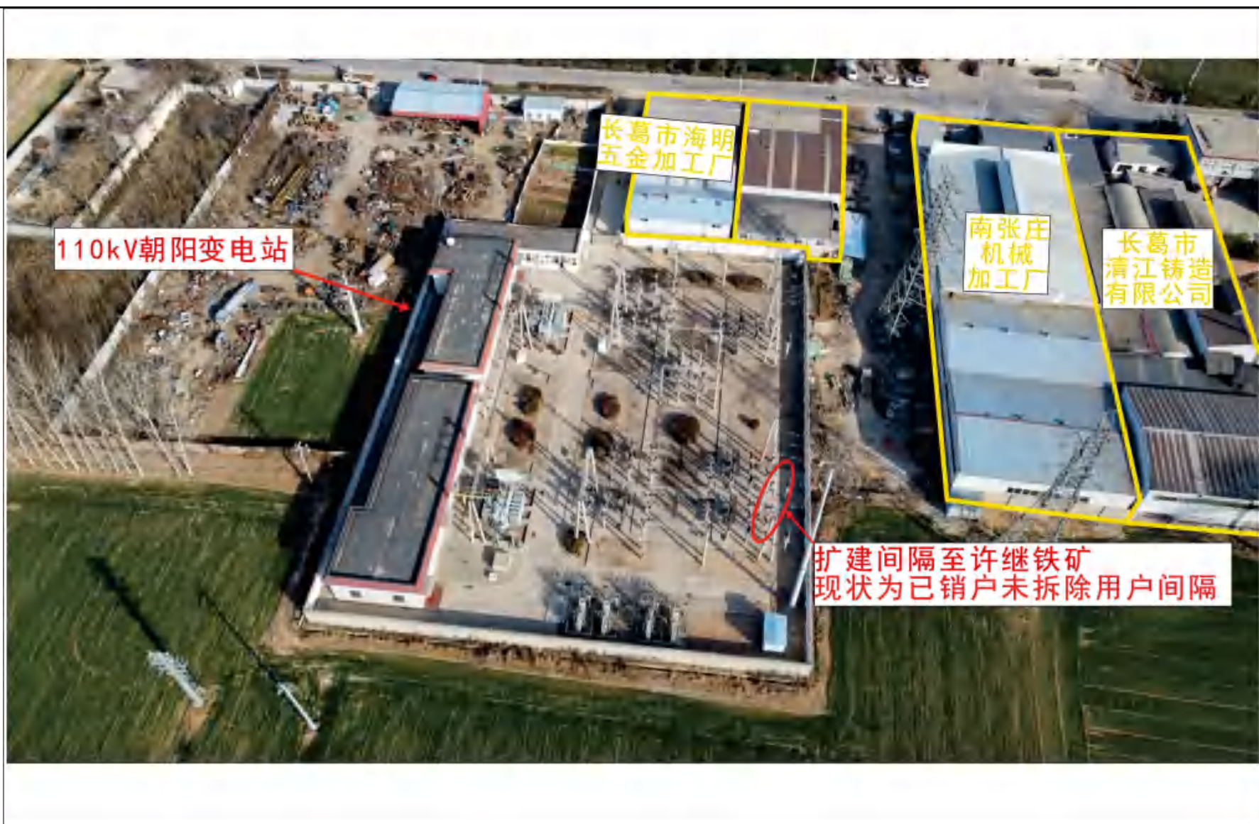
图 3-2-2 110kV 朝阳变电站间隔扩建侧现状照片
