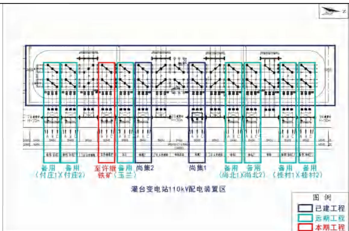
图2-6 本期灌台变电站110kV 间隔排列示意图
