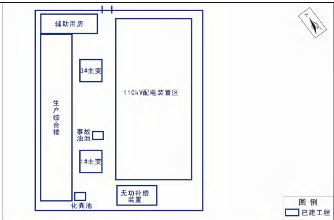
图2-7 110kV 朝阳变电站平面布置示意图
