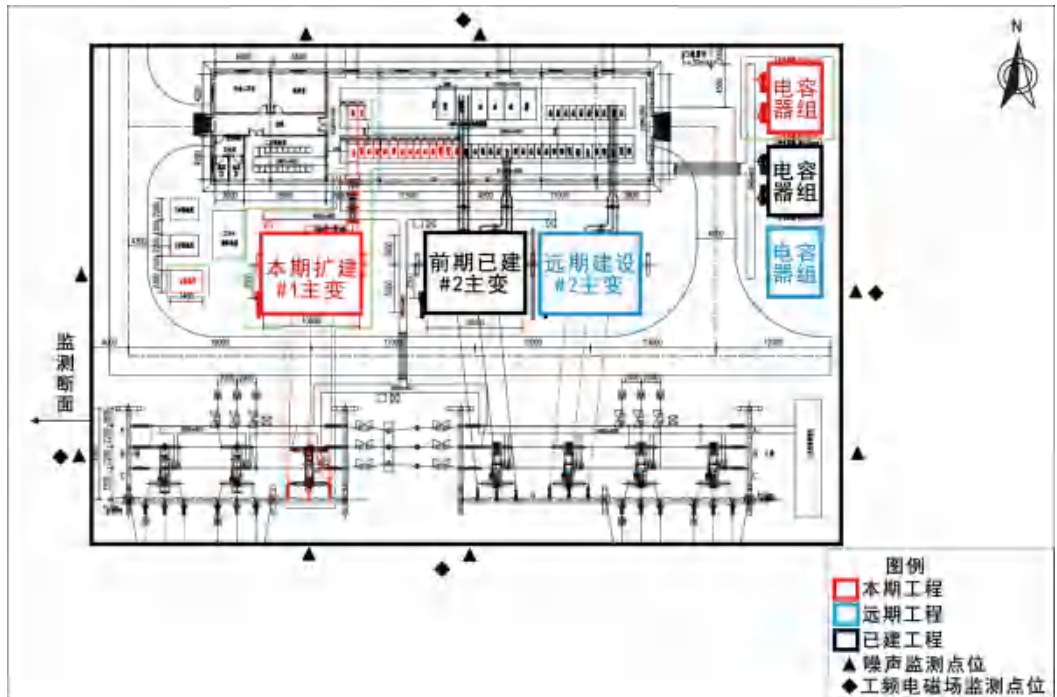
图 3-2 110kV 滨湖变电站监测点位示意图
