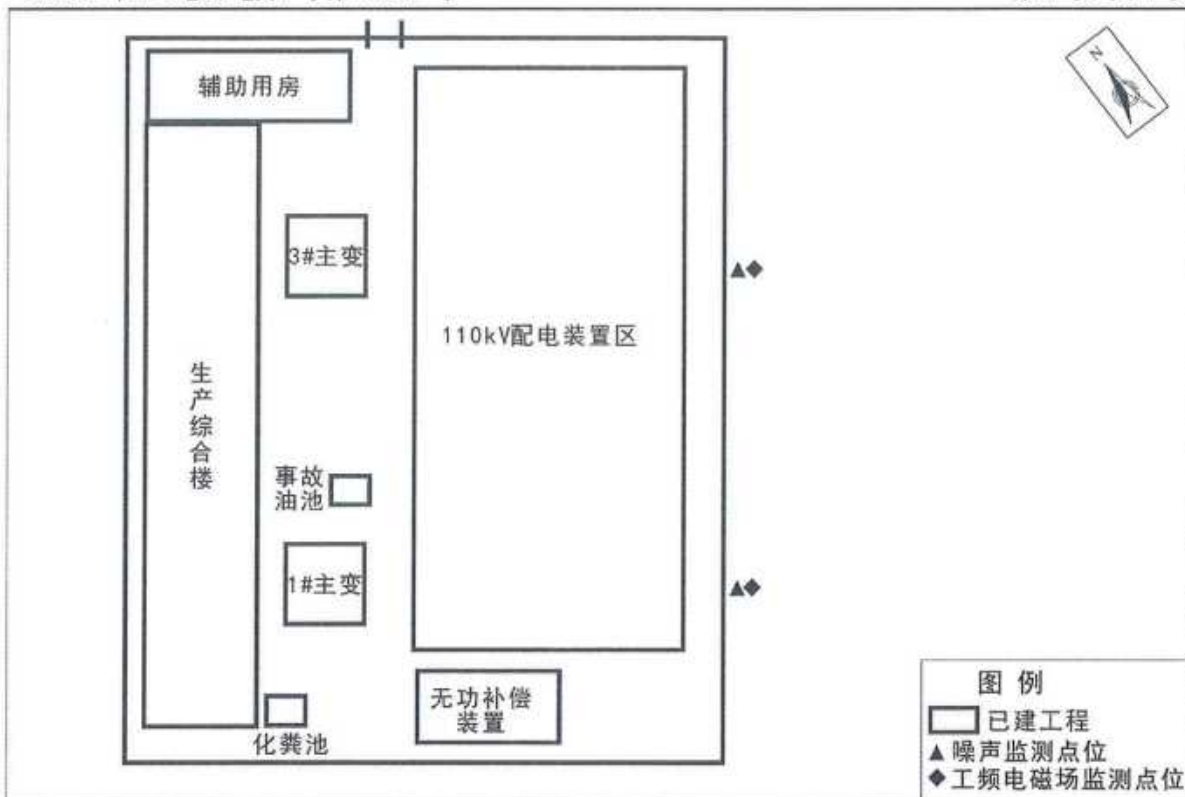
图 1-2 本项目朝阳变电站平面布置及监测点位示意图
