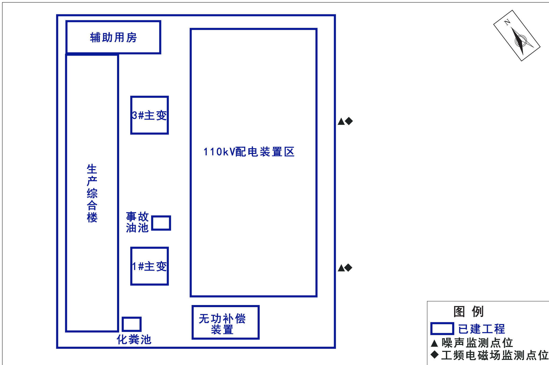
附图2-2 本项目110kV朝阳变电站平面布置及监测点位示意图
