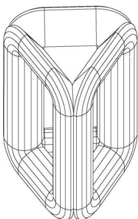
变压器铁心构造示意图
