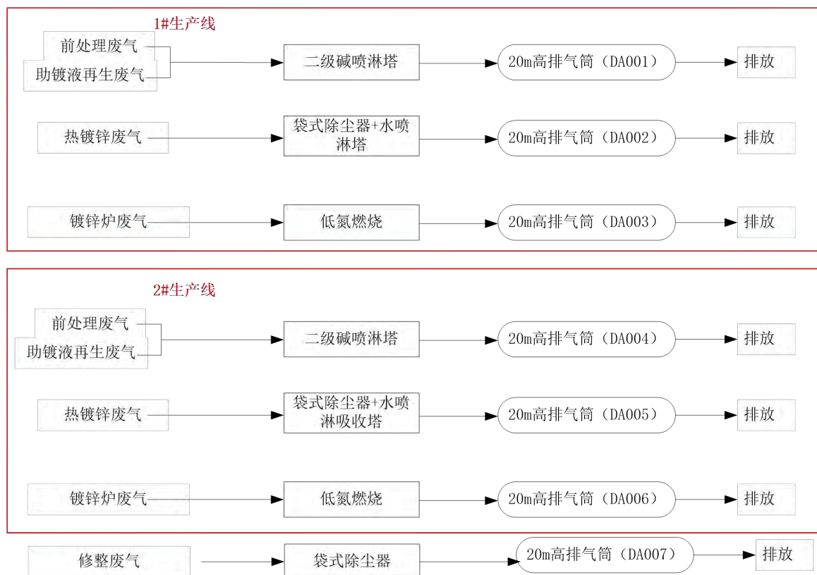
图 5.1-1 废气流向及处理措施示意图
