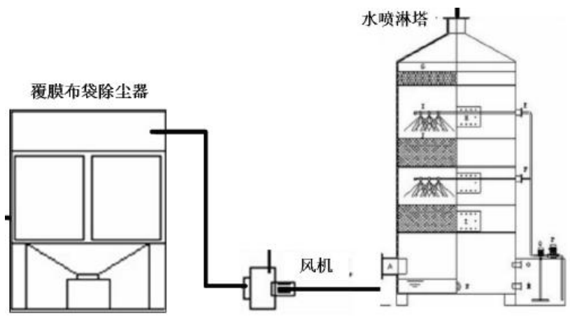
图 5.1-6 热镀锌废气治理工艺流程图
