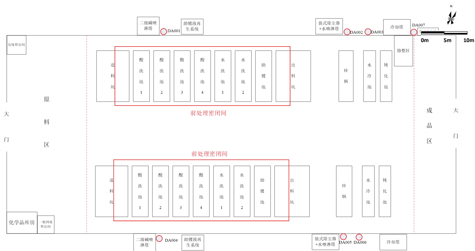
附图 5 车间内平面布置图
