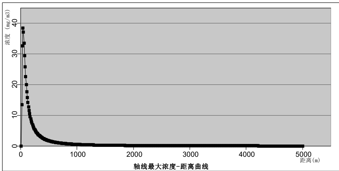
图 4.8-3 最不利气象条件下氨浓度随距离的变化曲线图
