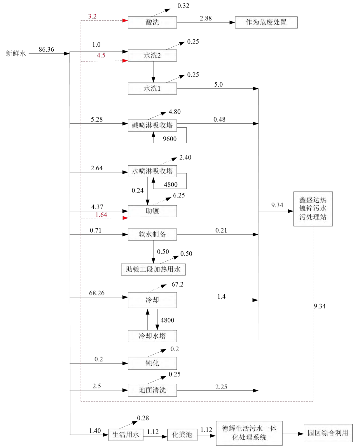
图 2.2-6 水平衡图 单位 m³/d
