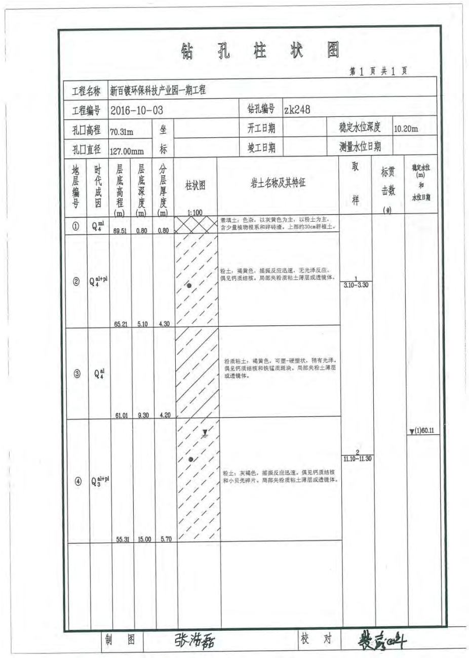
图 4.4-2 评价区钻孔柱状图
