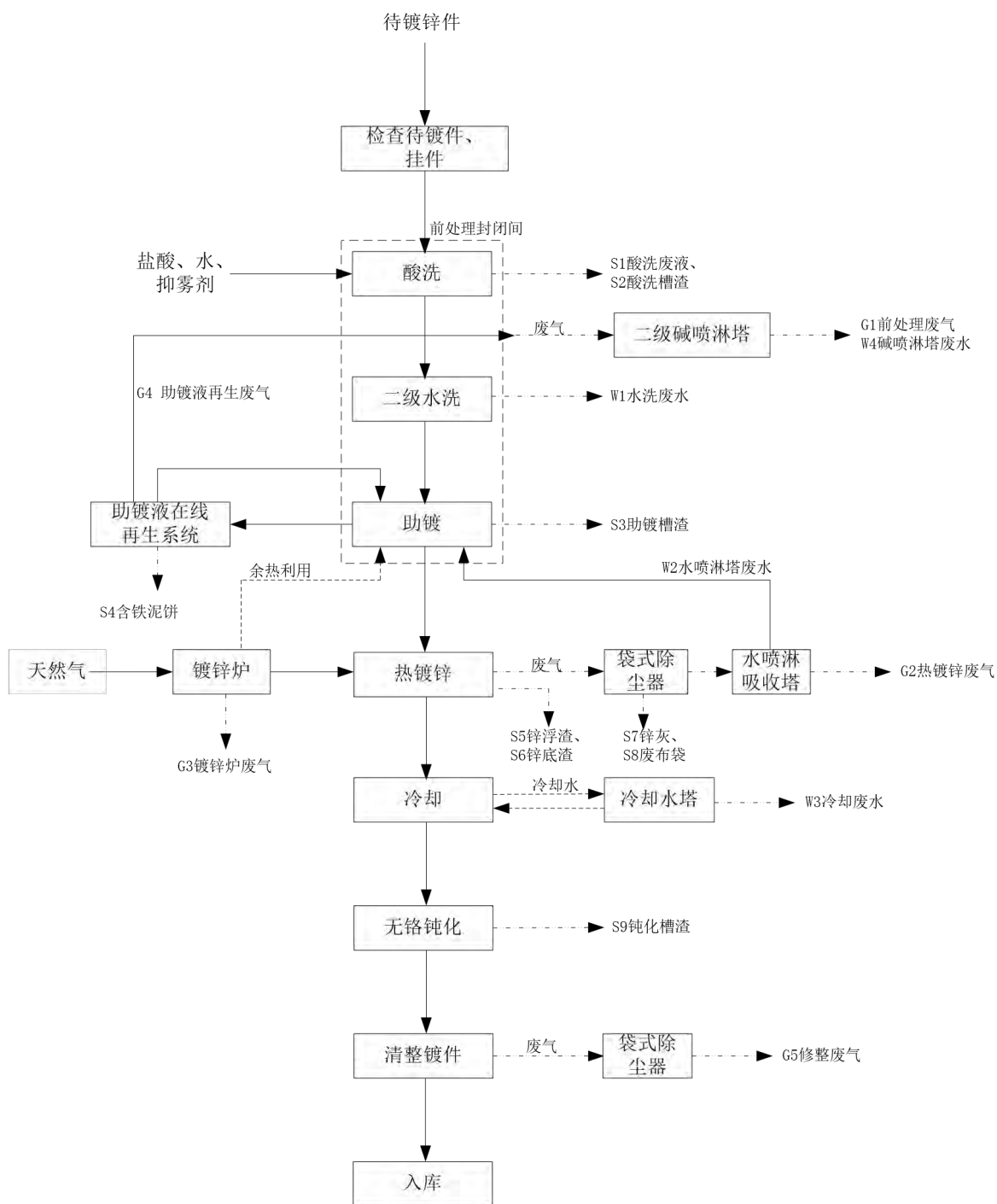
图 2.2-1 热镀锌生产工艺流程图
