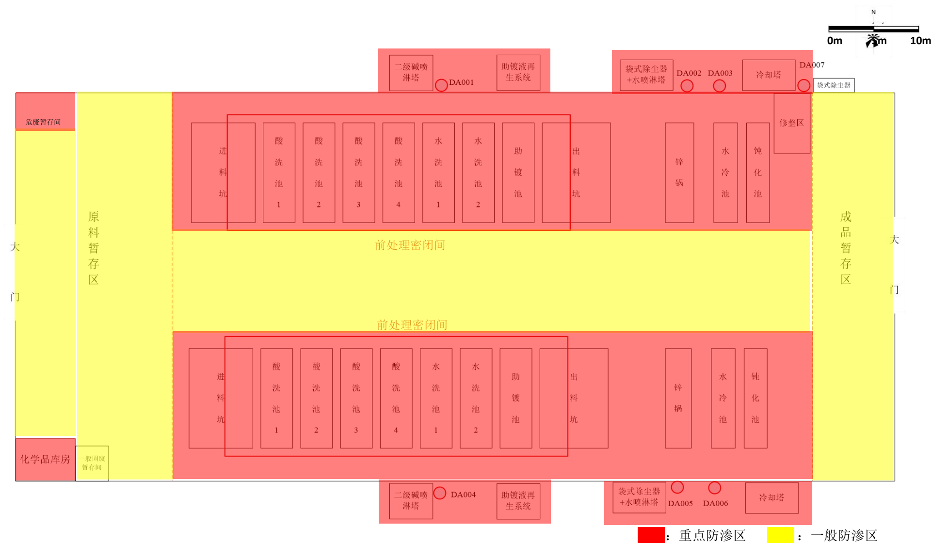
附图 6 车间内分区防渗图
