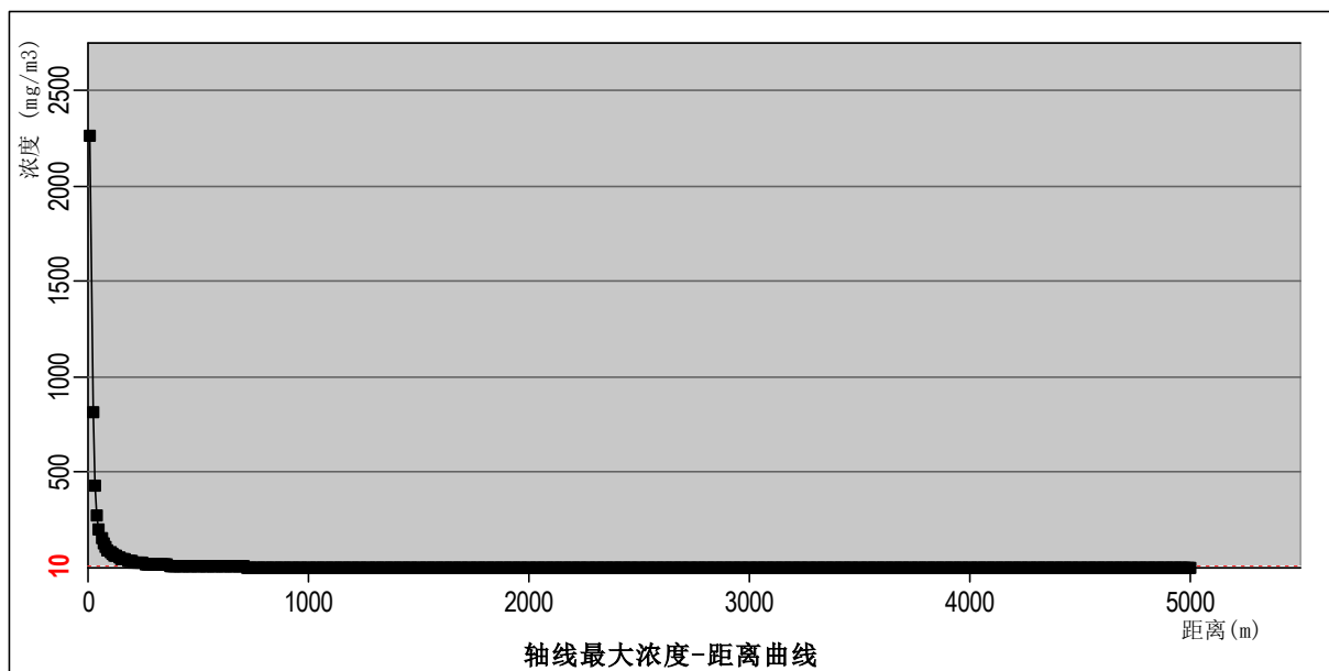
图 4.8-4 最不利气象条件下氯化氢浓度随距离的变化曲线图
