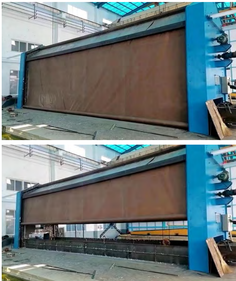
图 5.1-5 同行业企业锌锅封闭罩照片
