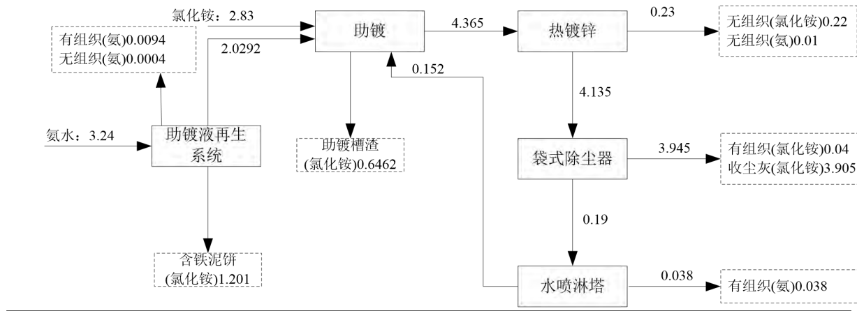
图 2.2-4 氨平衡图 单位 t/a
