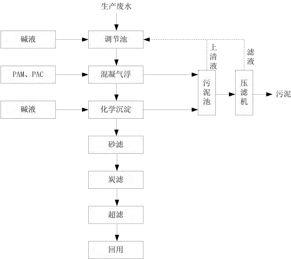
图 5.2-1 鑫盛达热镀锌污水处理站工艺流程
