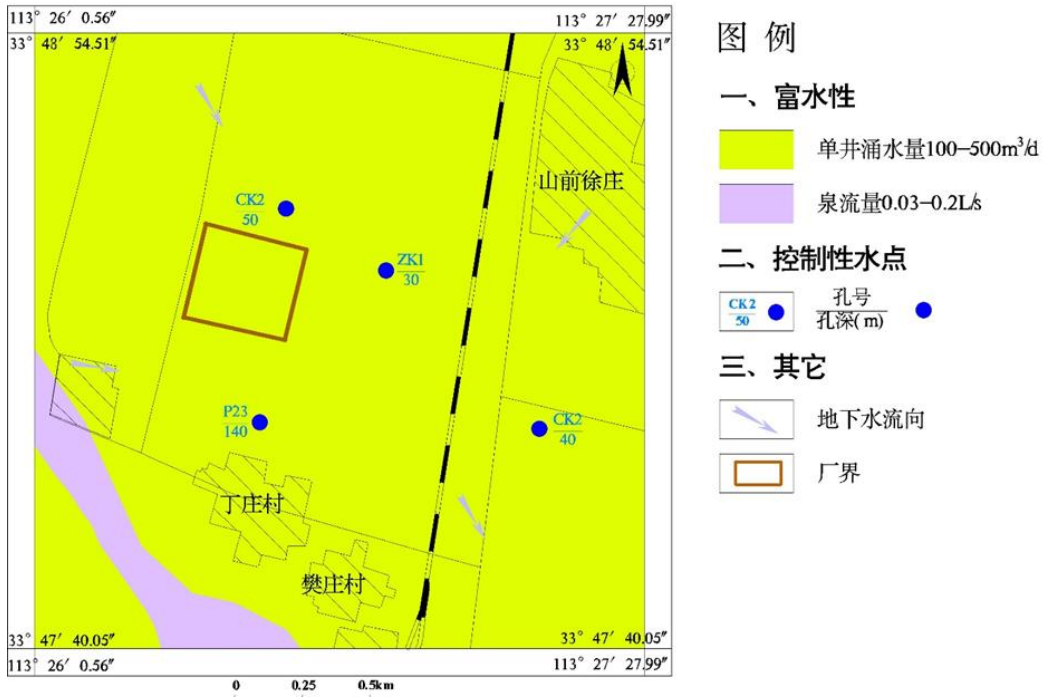
图 5-24 水文地质勘探孔平面布置图
