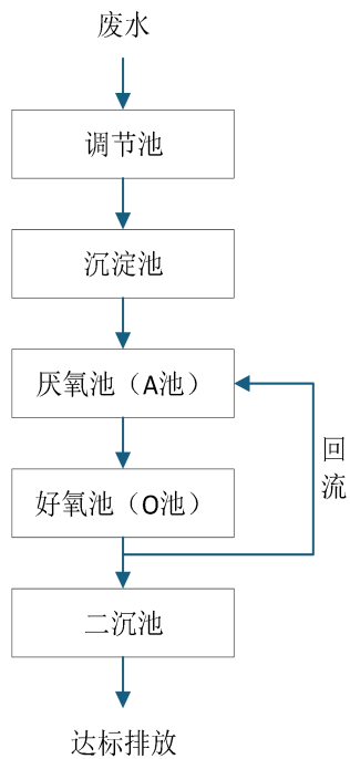
图 6-5 废水处理站工艺流程图
