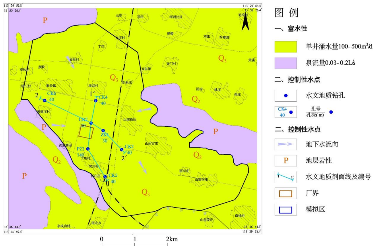
图 5-18 调查评价区水文地质图 (1:50000)
