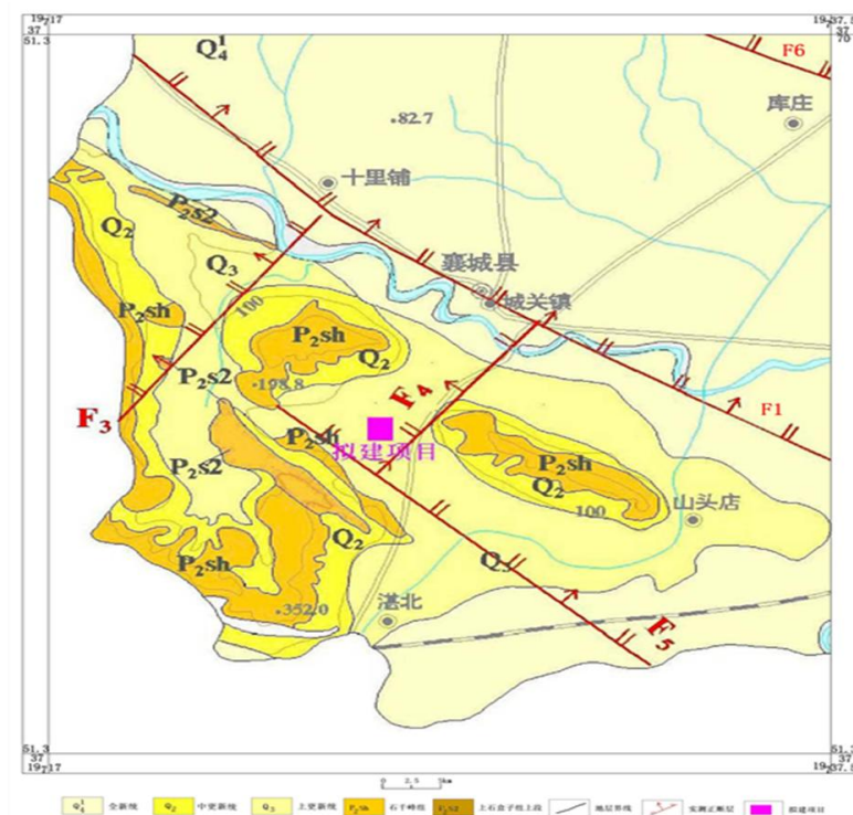
图 5-16 区域地层岩性及地质构造略图
