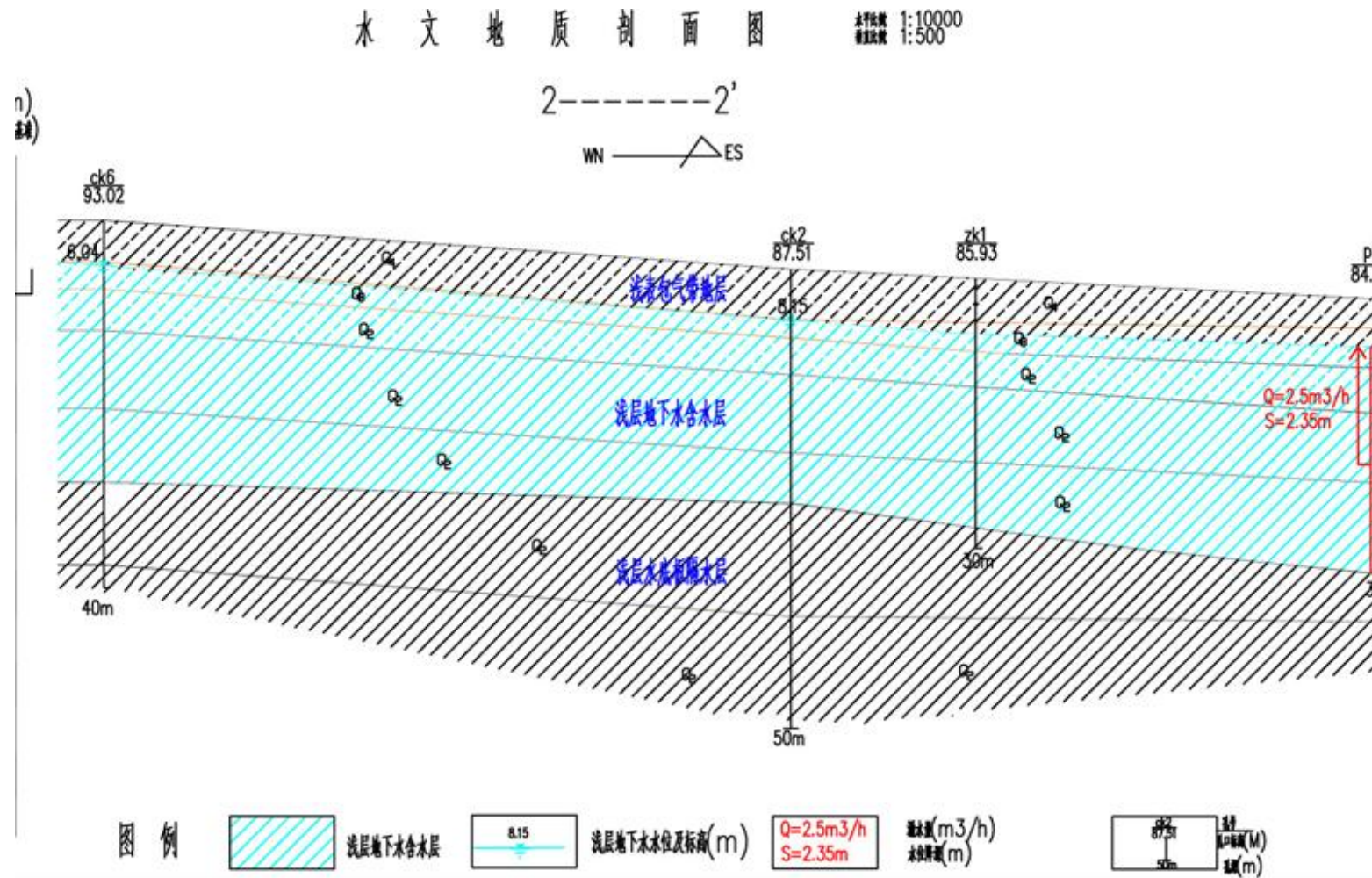
图 5-20 调查评价区 B-B' 水文地质剖面图
