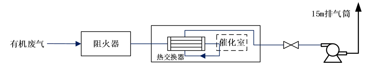
图 6-4 RCO 处理装置示意图
