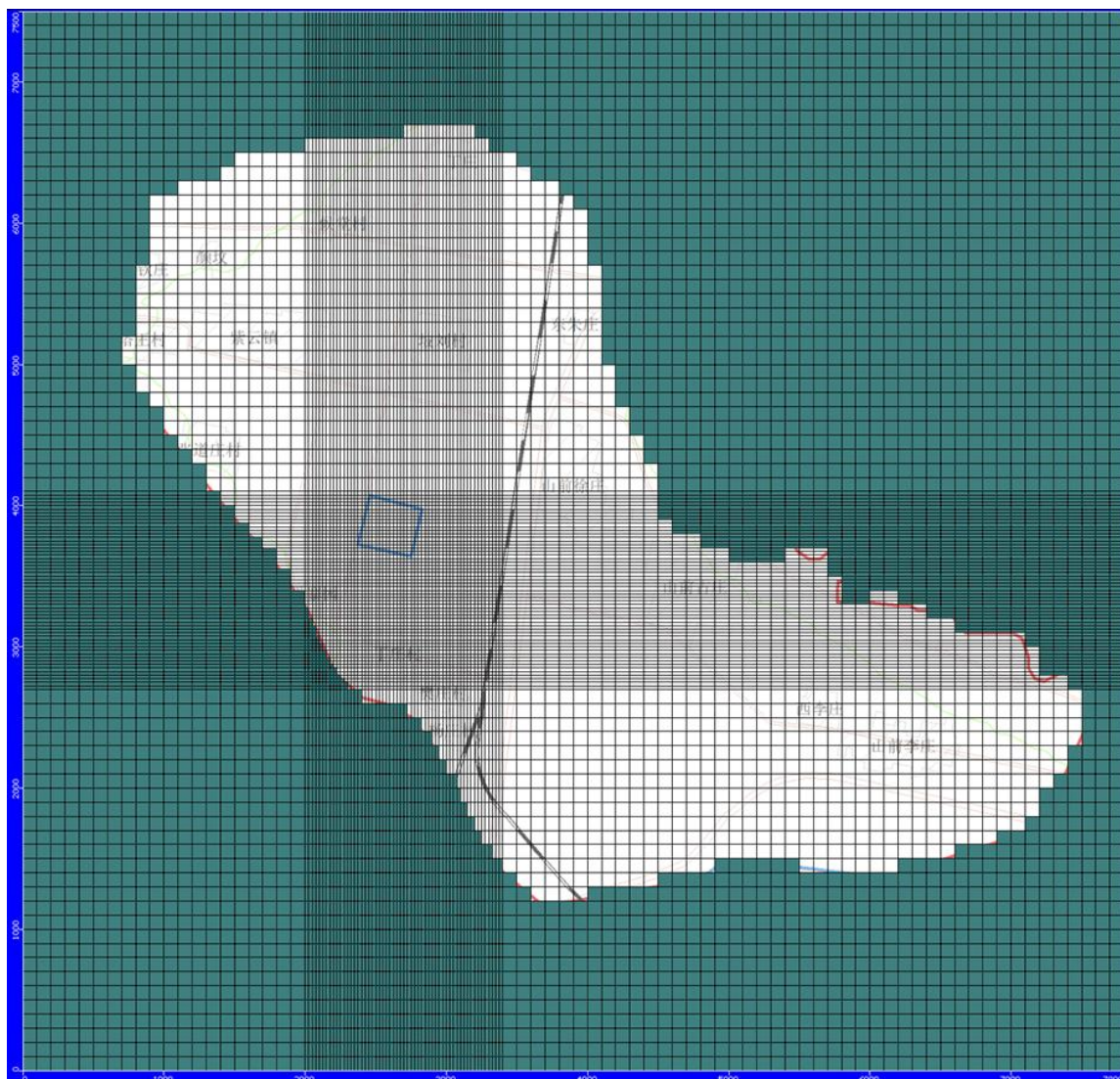
图 5-27 网格剖分
