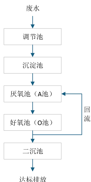
图 5-13 本项目废水处理站工艺流程图
