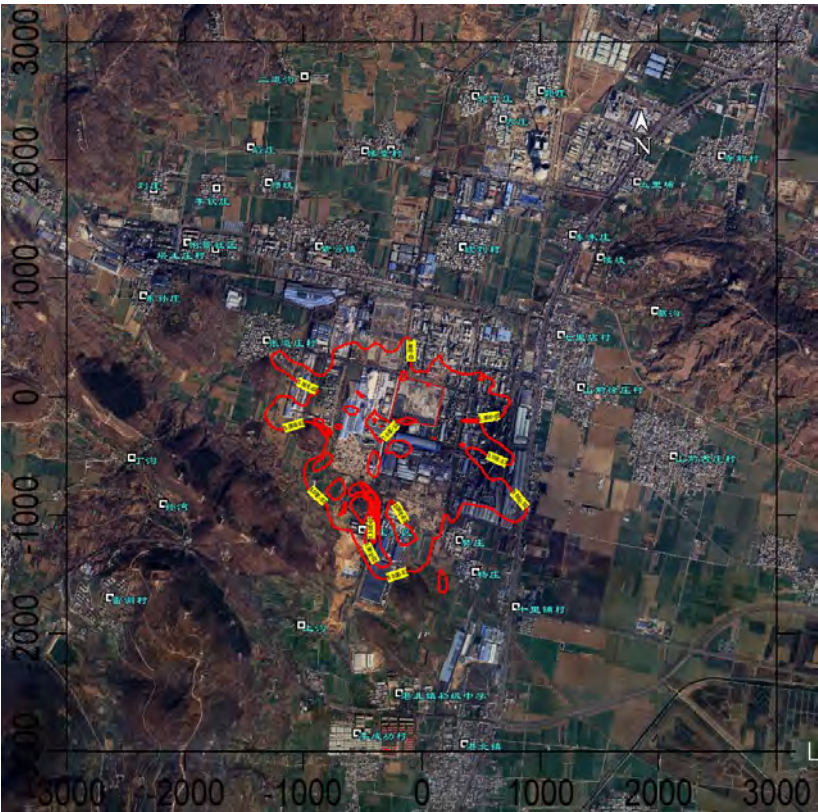
图 5-10 评价范围内甲醇日平均浓度叠加值分布图 \text{mg}/\text{m}^3
