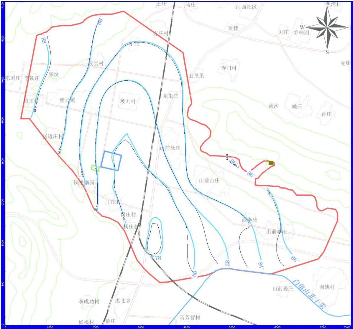
图 5-26 模型识别期流场拟合图
