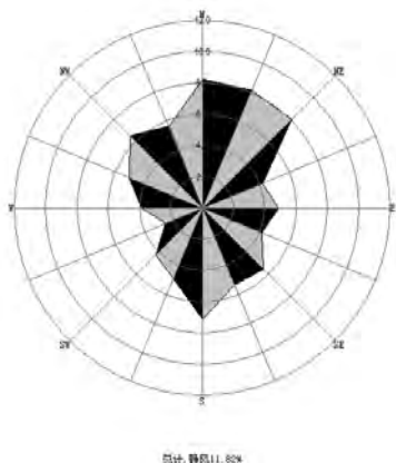
图 5-2 评价所在区域风频玫瑰图
