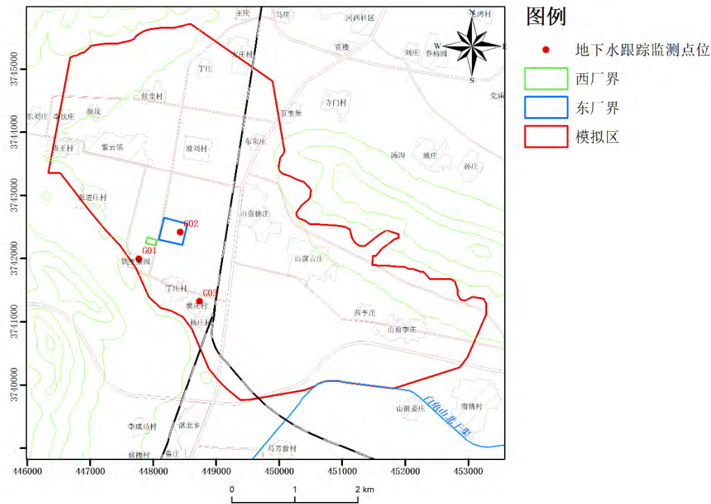
图 6-6 地下水水质跟踪监测点位置
