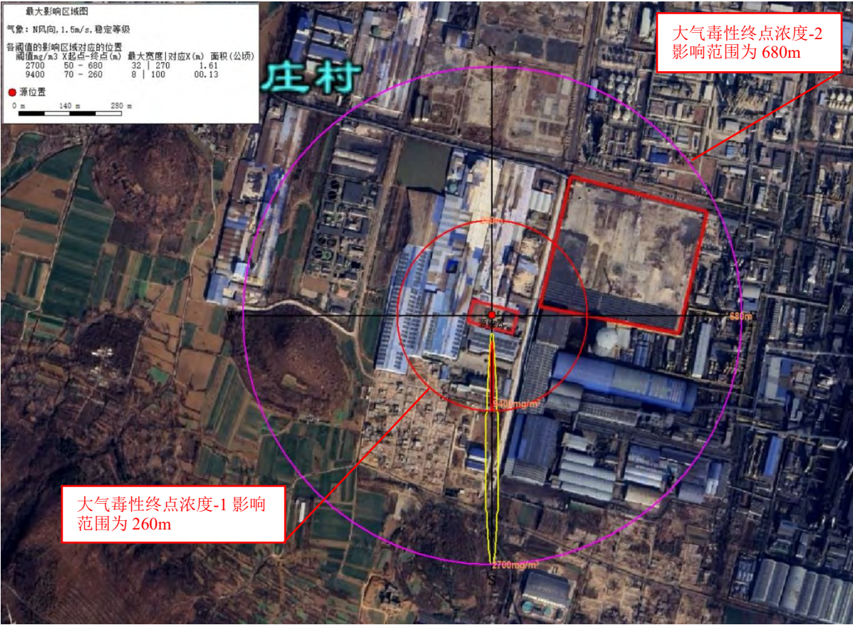
图 7-4（最不利）酯交换反应釜出料管线泄漏事故（甲醇）最大影响范围示意图
