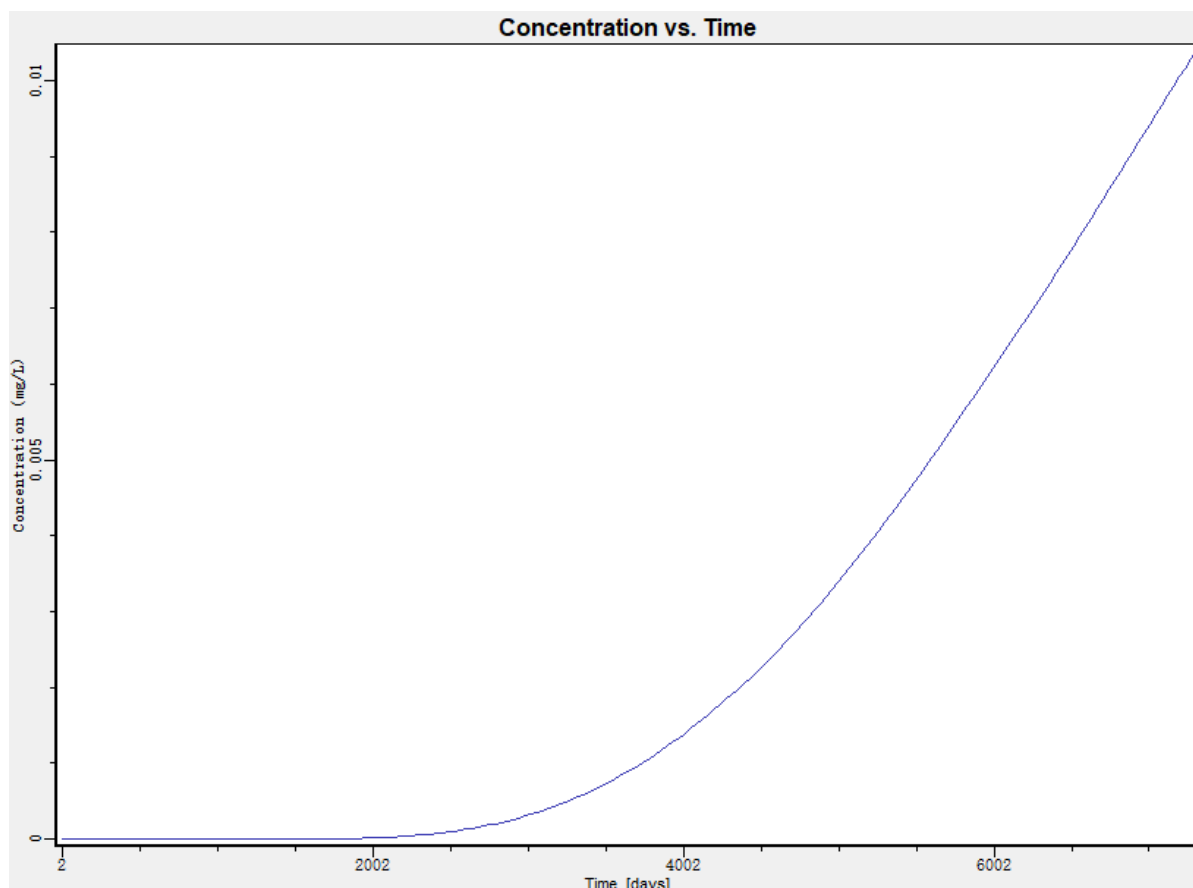
图 5-29 厂界监测点污染物（石油类）浓度随时间变化曲线
