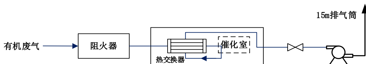
图 6-2 RCO 处理装置示意图
