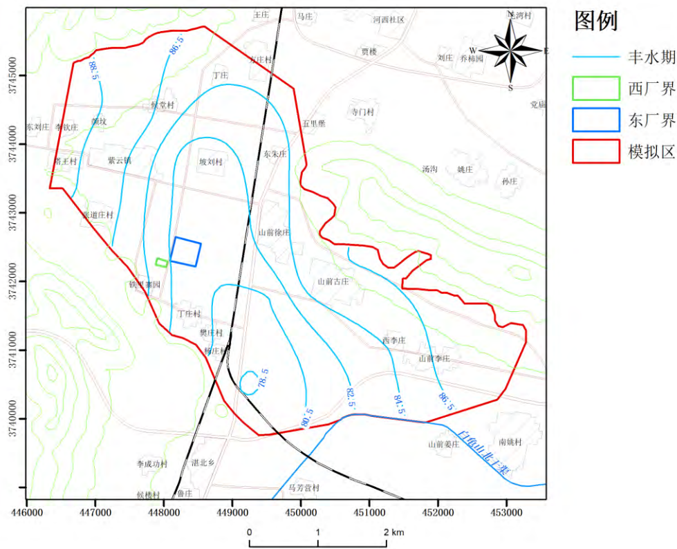
图 5-19 调查评价区浅层地下水流场图（丰水期）
