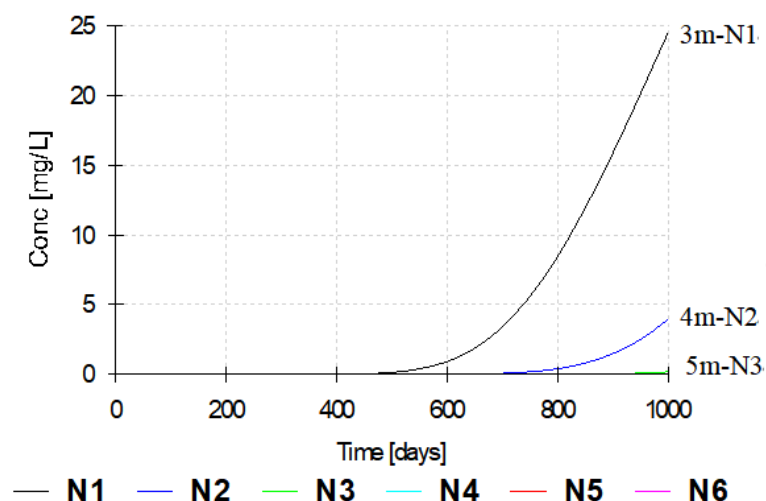
图 5-31 石油类浓度—时间曲线图
