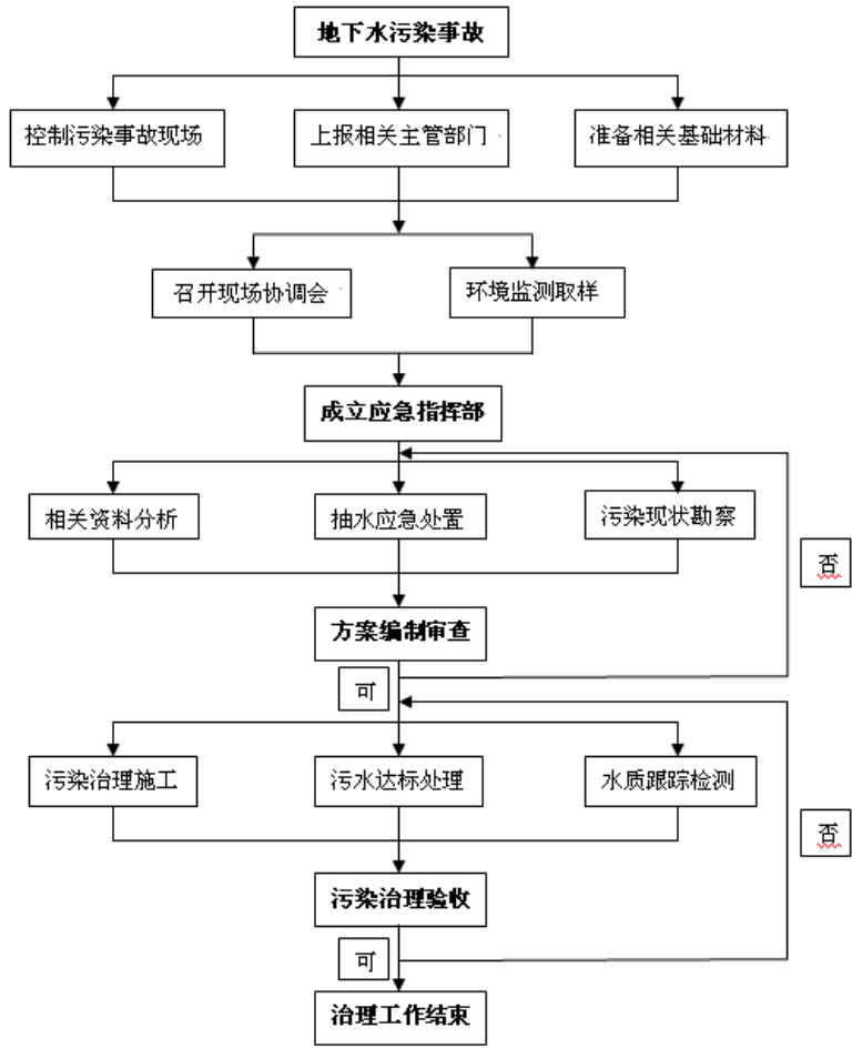
图 6-7 地下水污染应急治理程序框图
