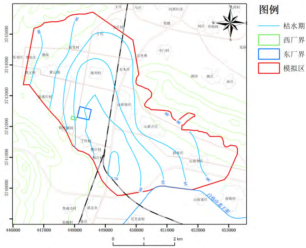
图 5-20 调查评价区浅层地下水流场图（枯水期）
