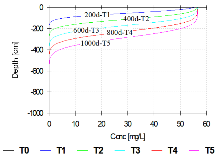
图 5-32 石油类浓度—深度曲线图
