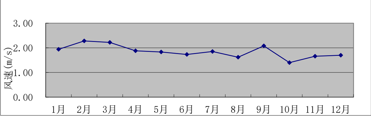
图 5-4 2024 年年平均风速月变化曲线图
