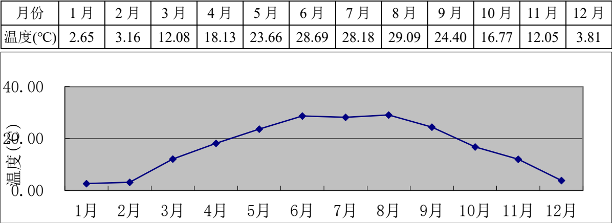
图 5-3 2024 年年平均温度的月变化图
