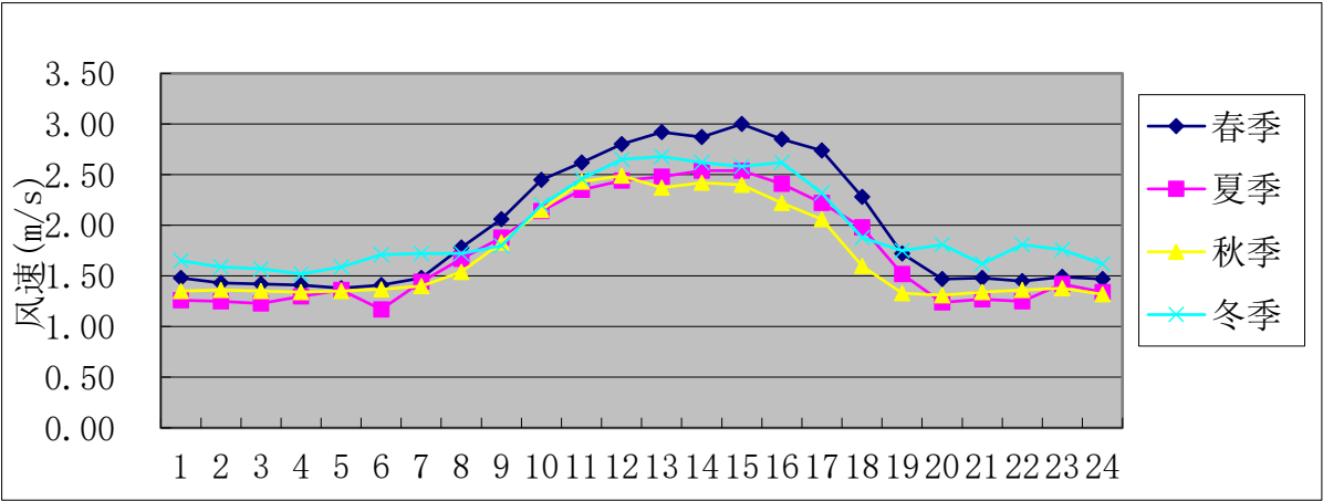
图 5-5 2024 年各季小时平均风速日变化曲线图
