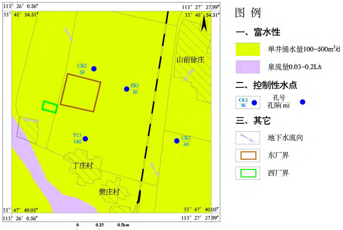
图 5-22 水文地质勘探孔平面布置图
