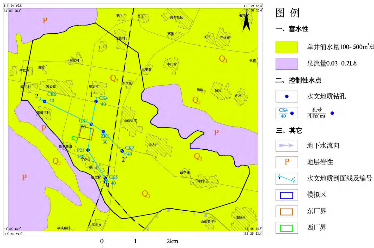
图 5-16 调查评价区水文地质图 (1:50000)
