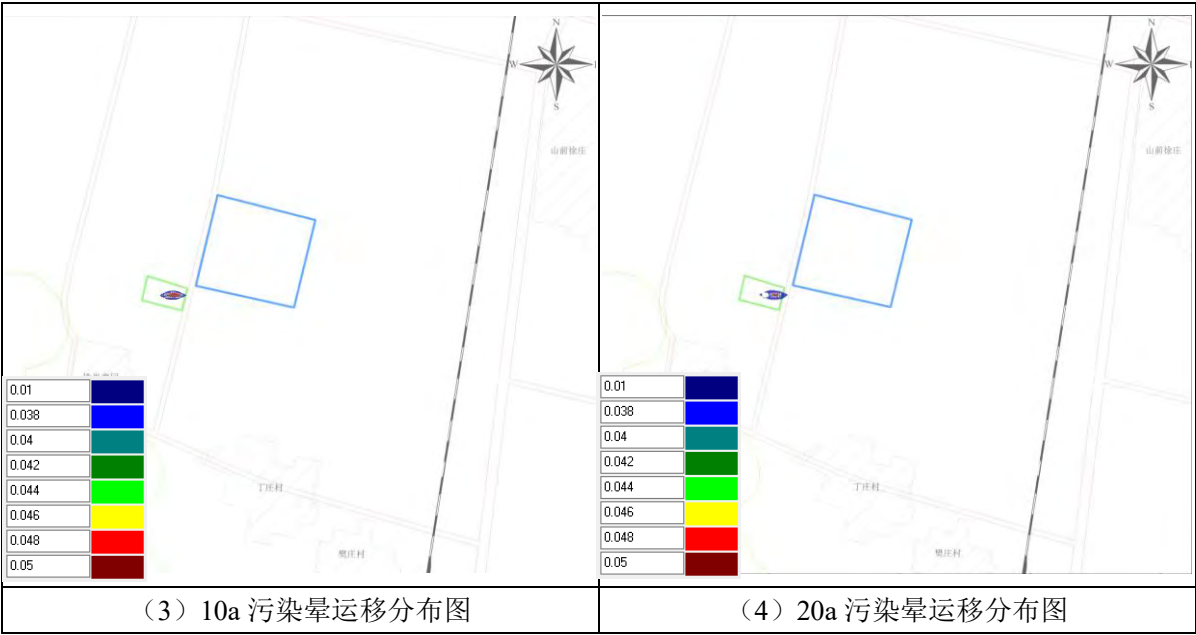
图 5-28 污染晕迁移分布图（石油类）
