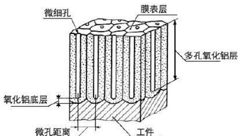
图 2.2-2 阳极氧化膜的结构示意图
