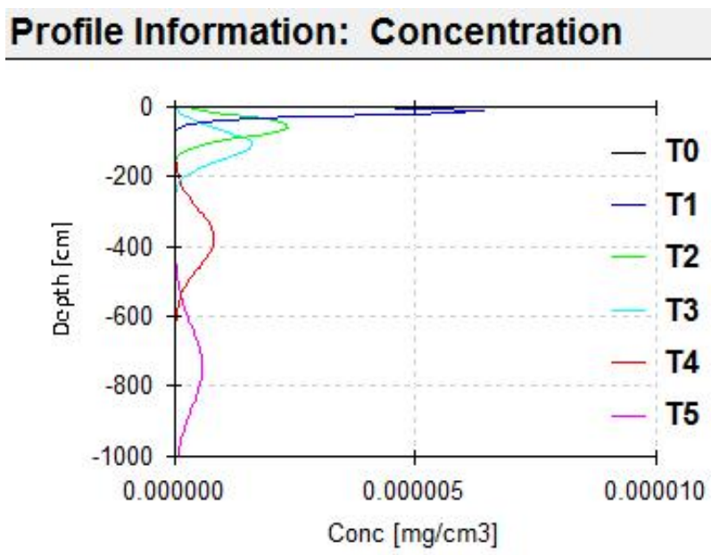
图 4.6-4 石油烃在不同时间沿土壤迁移情况
