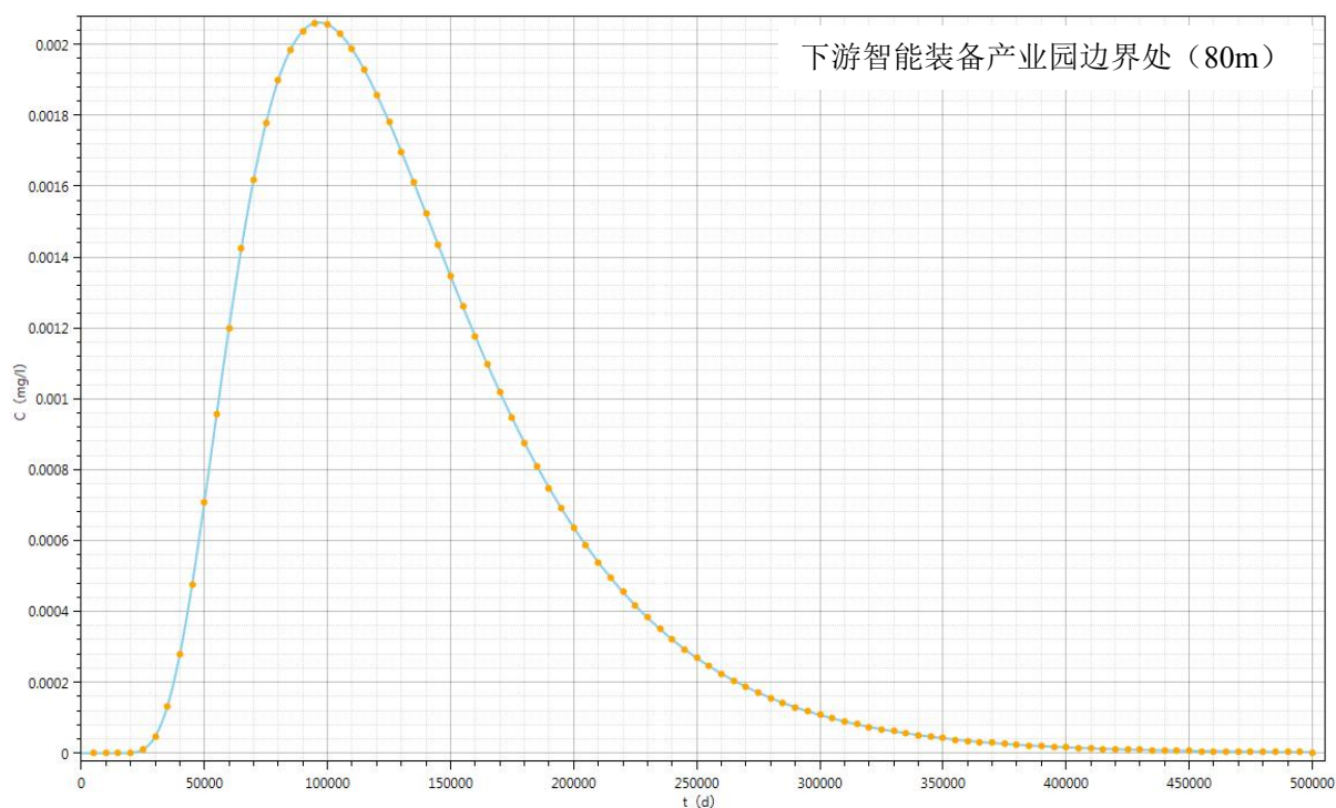
图 4.3-6 固定距离不同时间处铝浓度变化趋势
