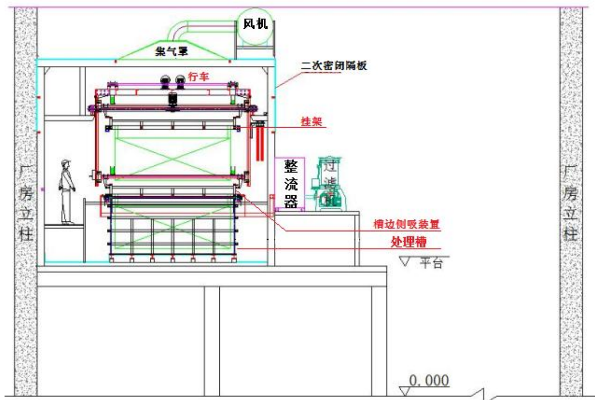
图 5.2-4 阳极氧化线封闭及酸雾废气收集示意图
