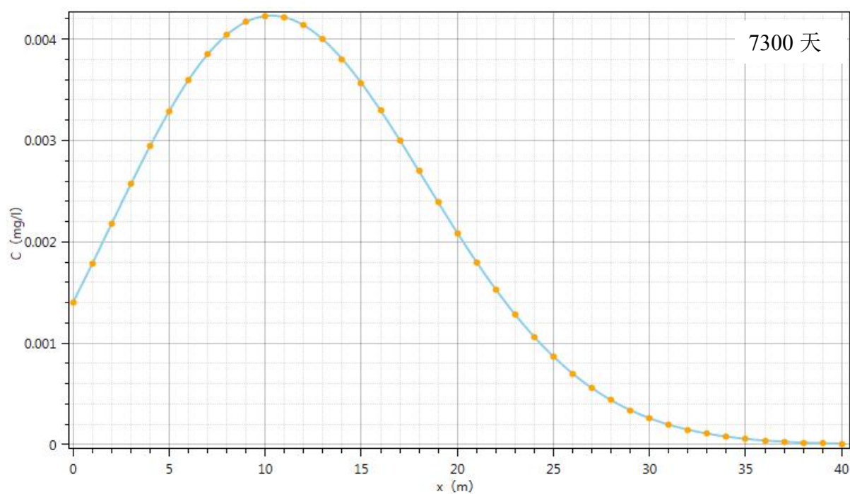
图 4.3-7 固定时间、不同距离硫酸盐浓度变化趋势
