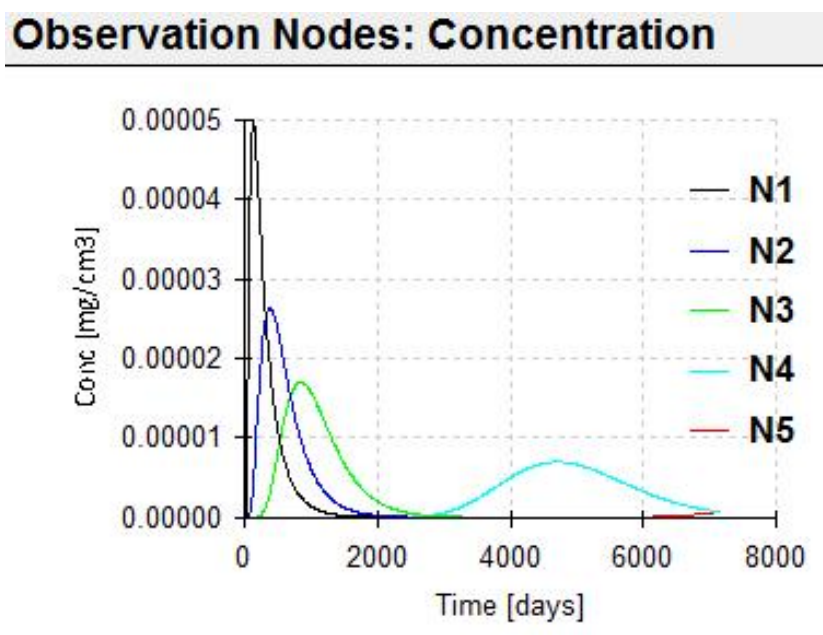
图 4.6-1 土壤不同深度总氟化物浓度-时间曲线
