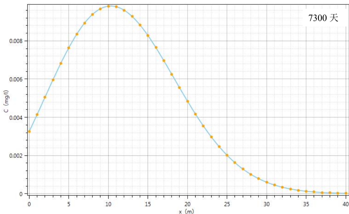
图 4.3-5 固定时间、不同距离铝浓度变化趋势
