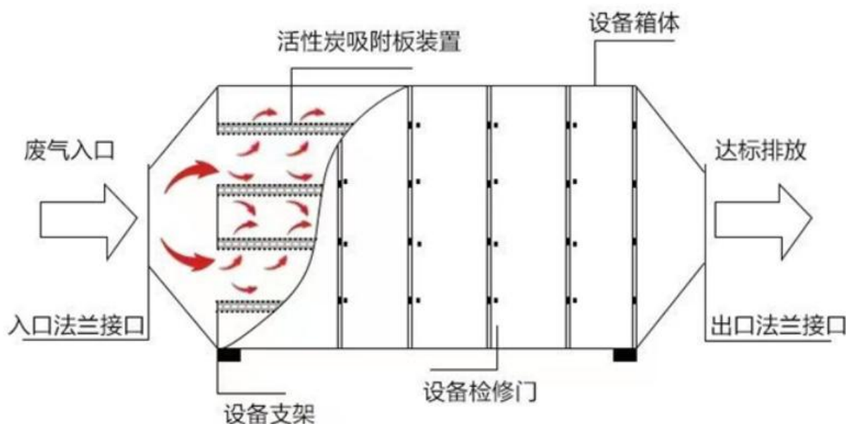
图 5.2-3 活性炭吸附装置工艺原理图
