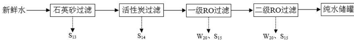
图 2.2-4 纯水制备生产工艺流程及产污环节示意图
