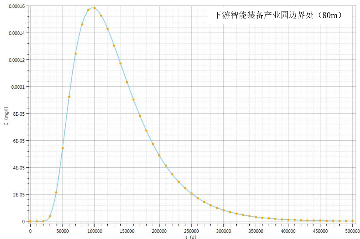
图 4.3-4 固定距离不同时间处总磷浓度变化趋势
