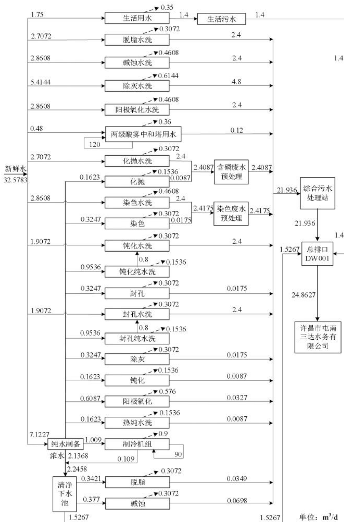
图 2.2-5 项目水平衡图
