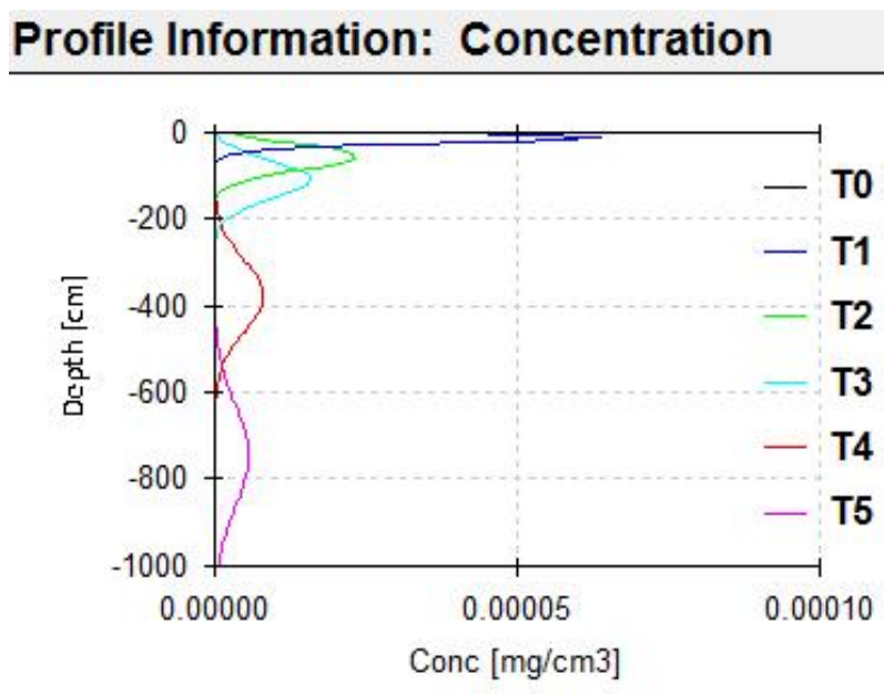
图 4.6-2 总氟化物在不同时间沿土壤迁移情况
