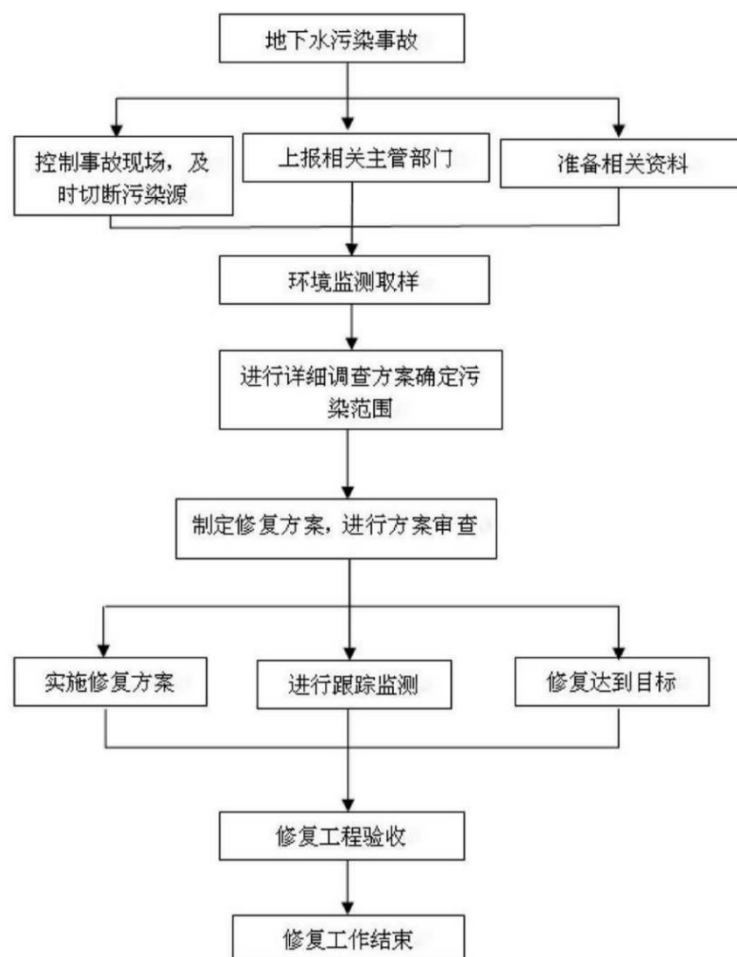
图 4.3-9 地下水污染应急治理程序框图
