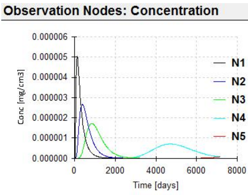
图 4.6-3 土壤不同深度石油烃浓度-时间曲线
