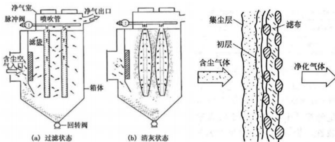
图 5.2-2 袋式除尘器工作原理图
