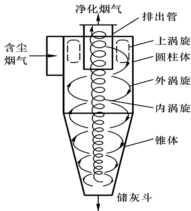
图 5.2-1 旋风除尘器工作原理图
