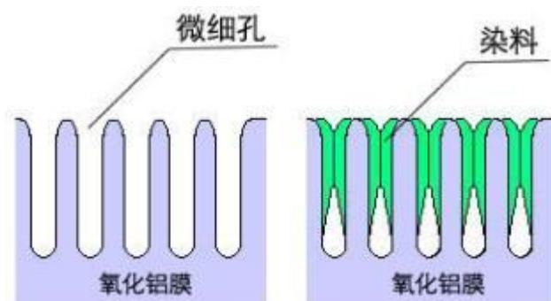
图 2.2-3 染色结构示意图
