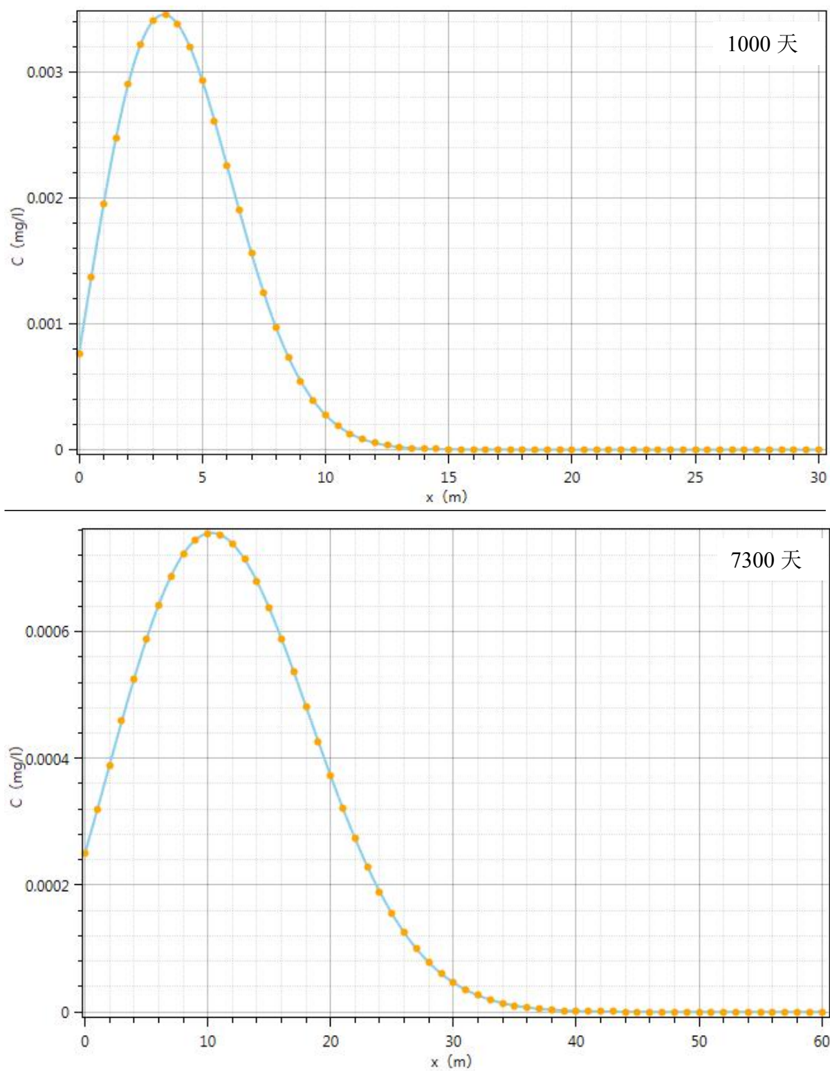
图 4.3-3 固定时间、不同距离总磷浓度变化趋势
