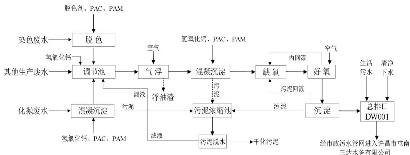
图 5.1-1 污水处理工艺流程图
