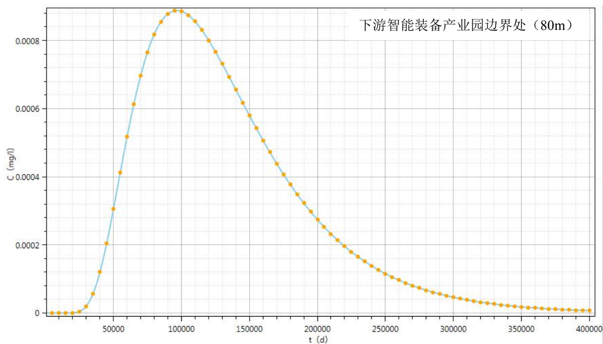
图 4.3-8 固定距离不同时间处硫酸盐浓度变化趋势
