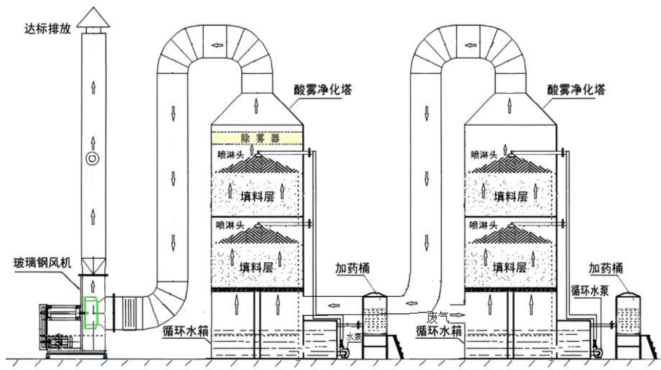
图 5.2-5 两级酸雾中和塔装置示意图
